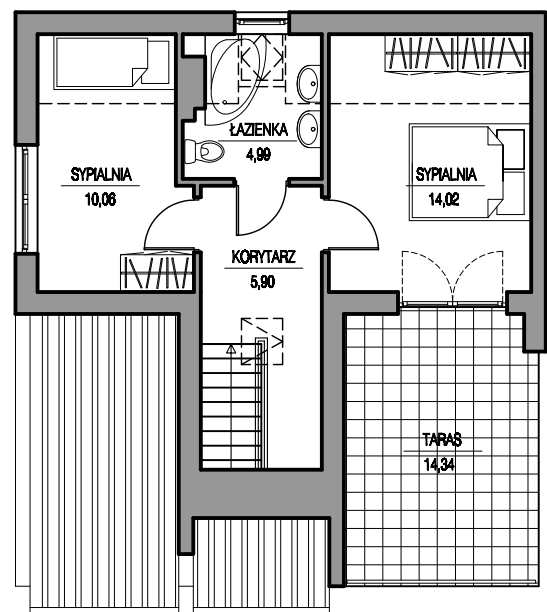
Poziom 2
